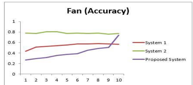
Fig. 13: Fan (Accuracy)
