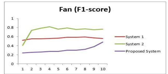
Fig. 14: Fan (F1-score)
