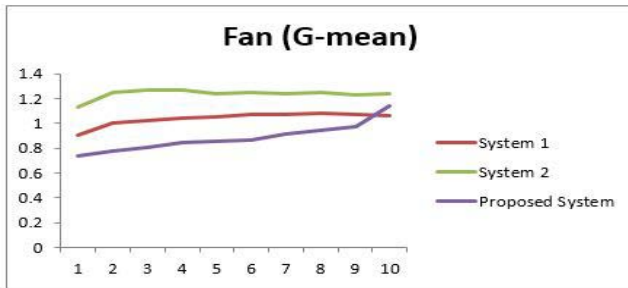
Fig. 15: Fan (G-mean)
